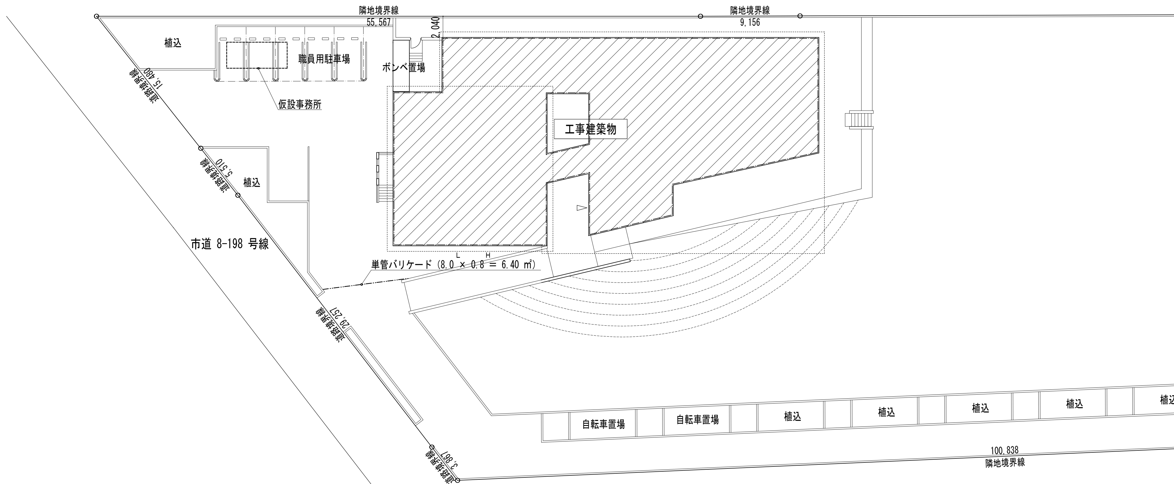
仮設計画図 (案) 1/200
