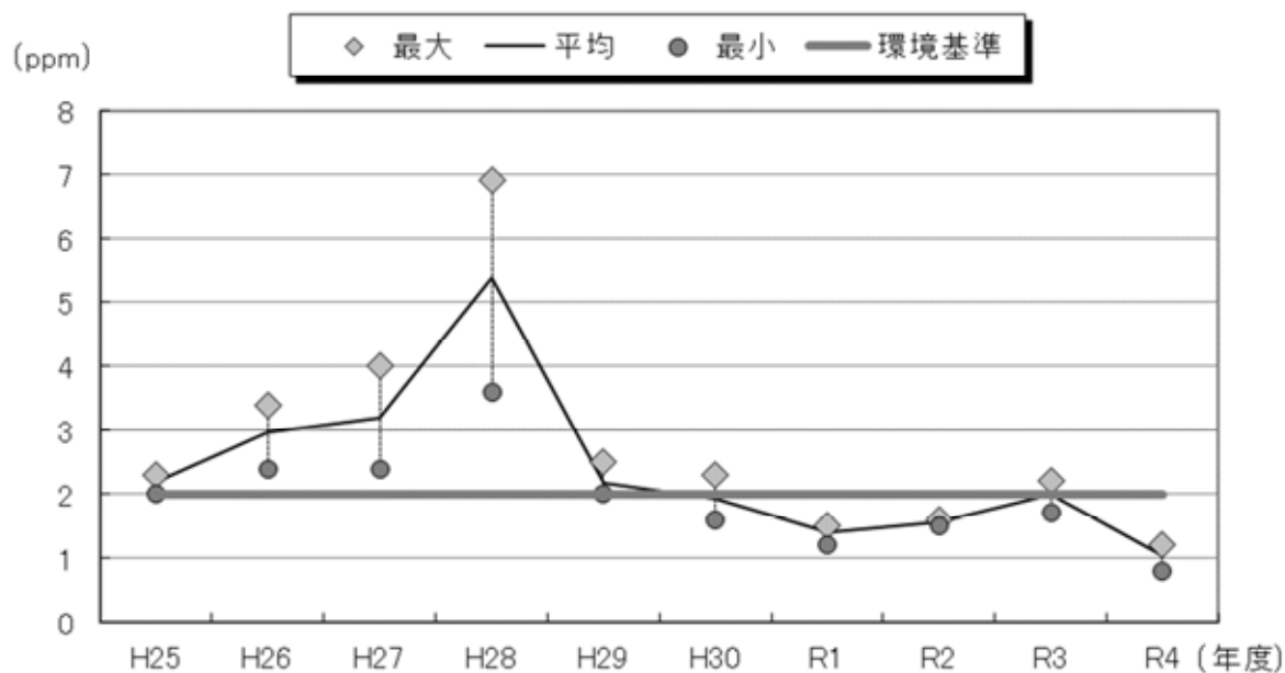
図 2-15 鹿島灘海域 (COD)
