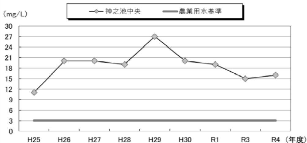
図 2-18 神之池 (COD)
