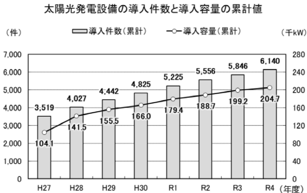
図 2-3 令和 5 年 3 月末時点までの太陽光発電設備 FIT 導入件数と導入容量の累計値の推移
