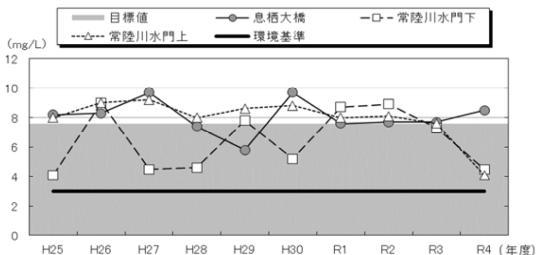
図 2-17 常陸利根川 (COD)
