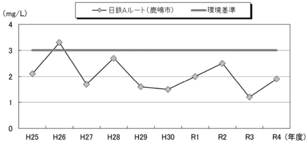
図 2-16 港湾北部 (COD)
