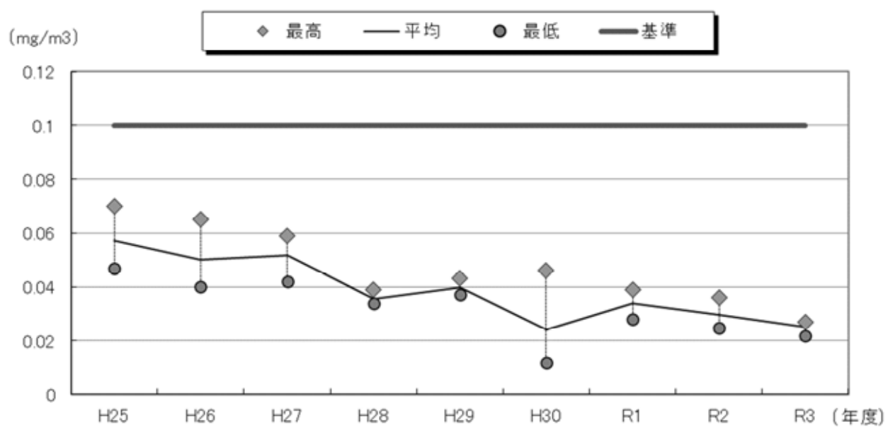
図 2-14 浮遊粒子状物質濃度の推移（2%除外値）(mg/m 3 )
