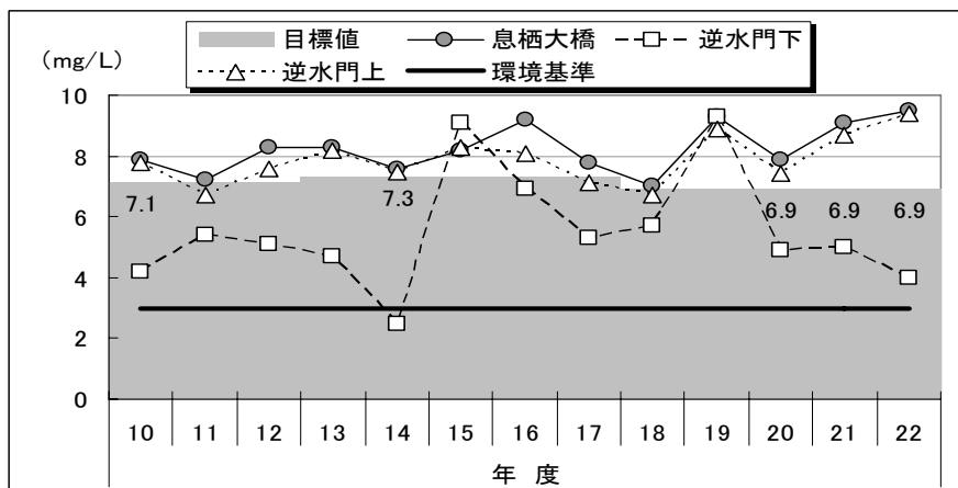
図7 常陸利根川におけるCOD*の推移
