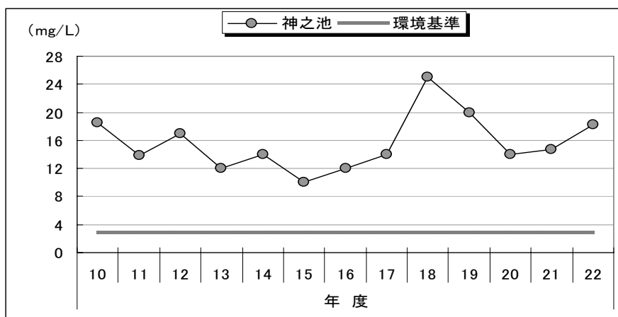
図6 神之池におけるCOD*の推移
