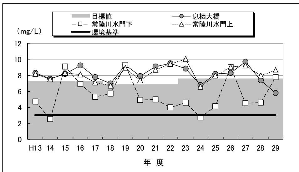
図 7 常陸利根川における COD の推移
