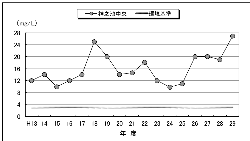
図 6 神之池における COD の推移
