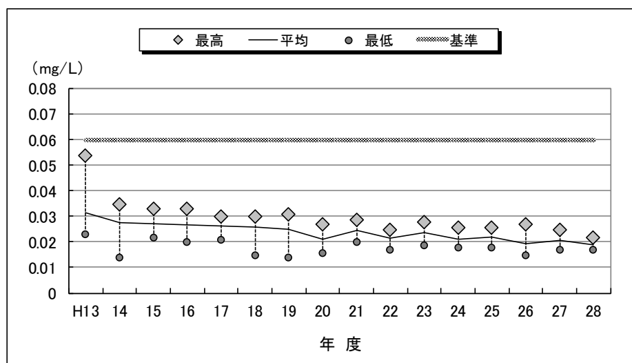
図2 二酸化窒素濃度の推移(98%値)
