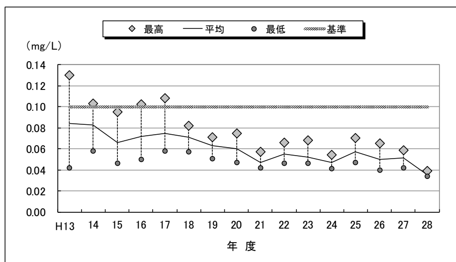
図3 浮遊粒子状物質濃度の推移(2%除外値)
