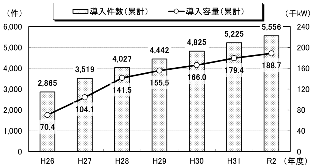
図 2-3 令和 3 年 3 月末時点までの太陽光発電設備 FIT 導入件数と導入容量の累計値の推移
