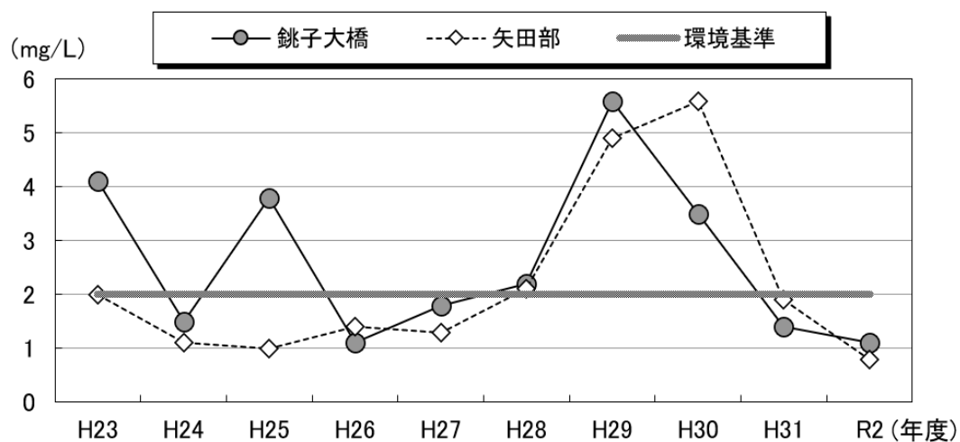
図 2-19 利根川下流 (BOD)
