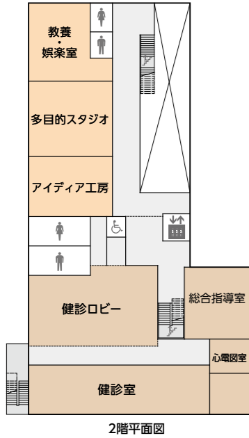
2階平面図
