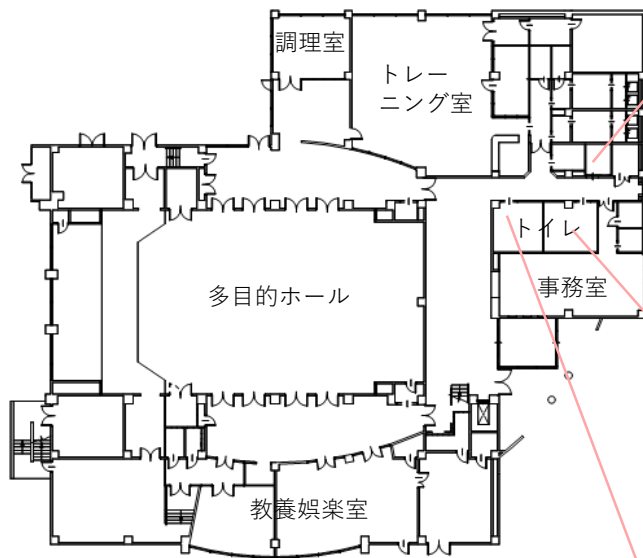
1 階平面図
