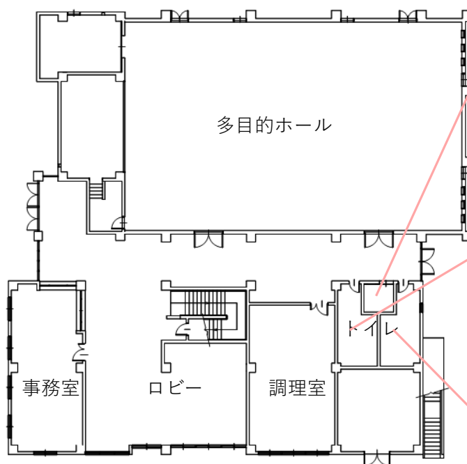
1 階平面図
