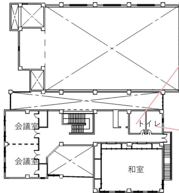
2 階平面図
