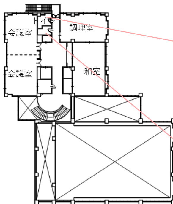
2 階平面図
